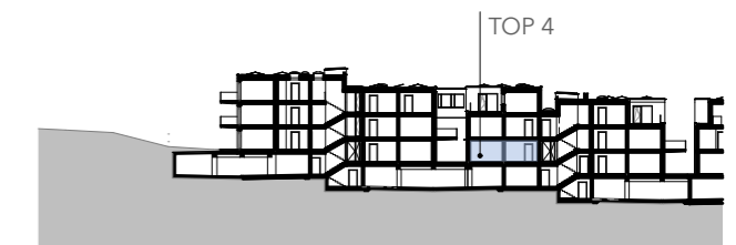
Übersicht Schnitt
